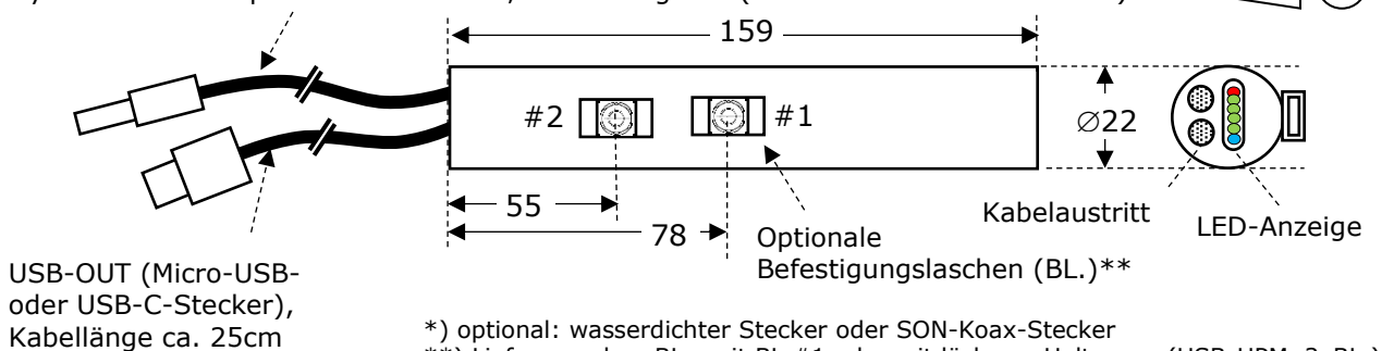
Bild 5: Abmessungen und Anschlüsse (nicht maßstabsgerecht, Maße in mm)
