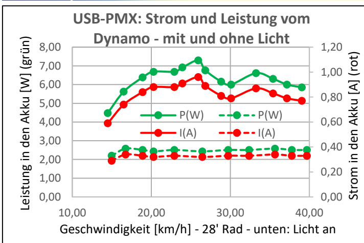
Bild 3: Ladestrom über der Geschwindigkeit mit und ohne Fahrradlicht, für einen typischen Nabendynamo (Shimano)
